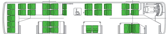
TNB 12 (4 doors)
